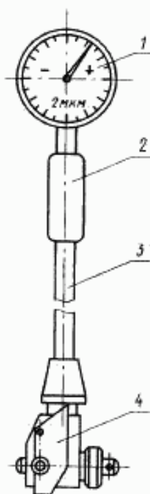
1 — отсчетное устройство; 2 — ручка; 3 — корпус; 4 — мостик.
